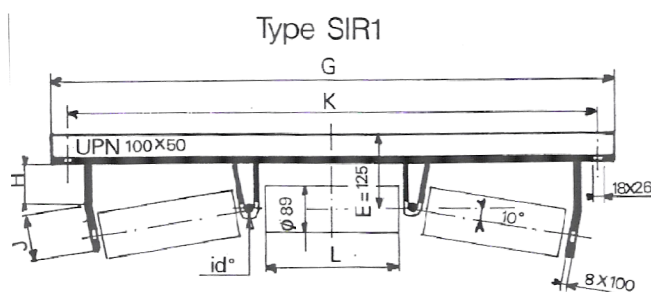
Pour rouleaux ø 89 (LM 204 Hy / PNE 53 300)
