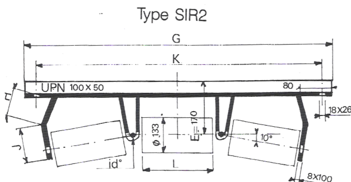
Pour rouleaux ø 133 (LM 204 Hy / PNE 53 300)
